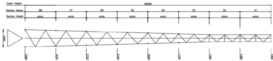
Principskitse for 48 meter gittermast (her lagt ned)
